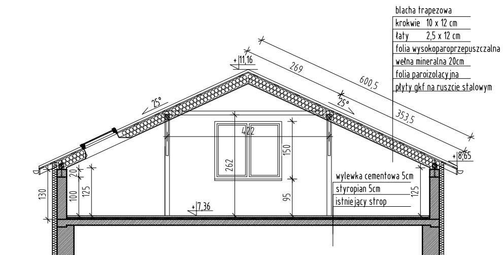
PRZEKRÓJ A-A
